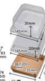
⑪ 蓋 ⑩ 蓋 ⑨ 本体 KM-75 (約310g)
